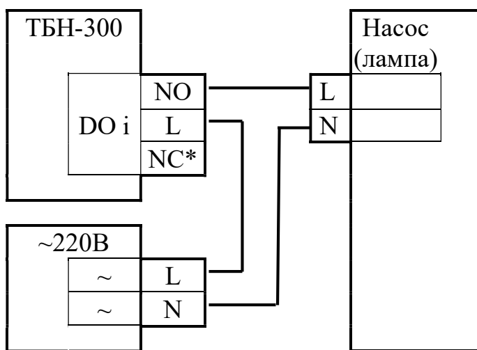
Рисунок 3.3 – Схема подключения реле включения насоса (без схемы контроля одновременного включения двух насосов) и ламп сигнализации, i – номер канала (1 – 10); * – контакт «NC» присутствует только на выходах DO1 – DO4 приборов серии 0001.
