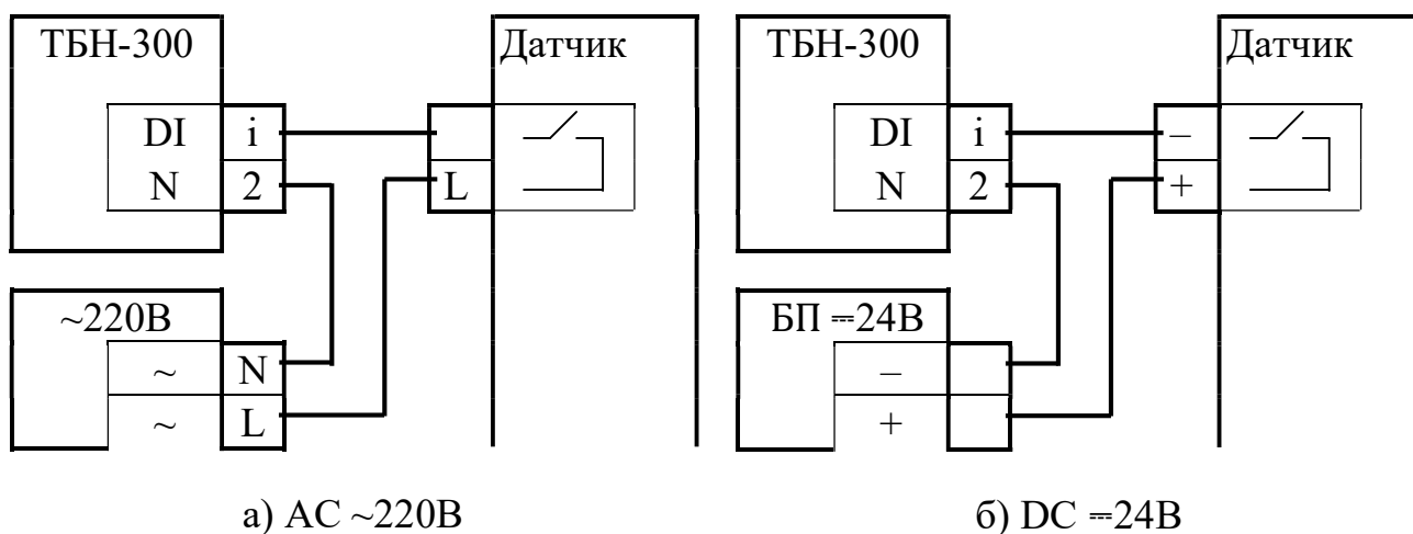
Рисунок 3.2 – Схема подключения датчика типа «сухой контакт»
